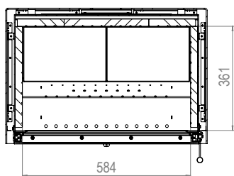
PRZEKRÓJ A-A
